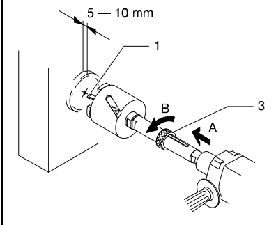
Bohrkronenschaft ohne Absaugglocke Bild 6
