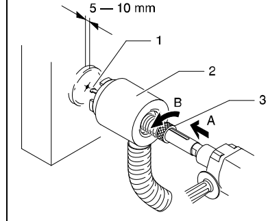
Bohrkronenschaft mit Absaugglocke Bild 7
