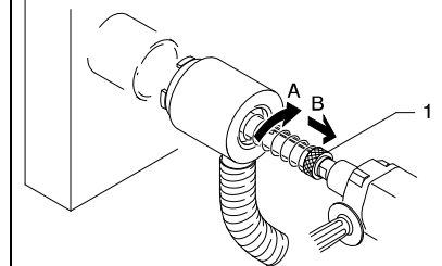
Bohrkronenschaft mit Absaugglocke Bild 9
