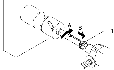
Bohrkronenschaft ohne Absaugglocke Bild 8
